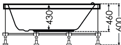
Seitenansicht mit fertig vormontierten Untergestell +/-
